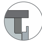
Gola piatta con presa "Step" Flat "Step" handle grip for flat groove
